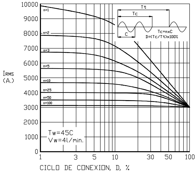
Corriente I_{RMS} máxima según el ciclo de trabajo.
