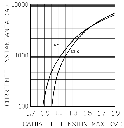
Características de conducción.
