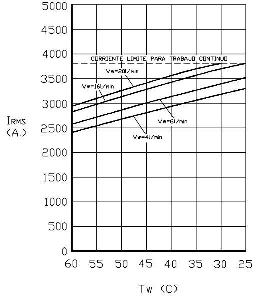
Corriente I_{RMS} máxima en trabajo continuo.
