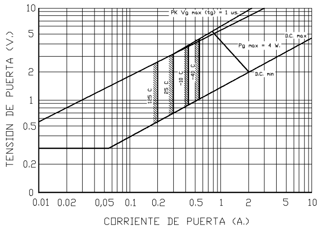
Características de puerta.
