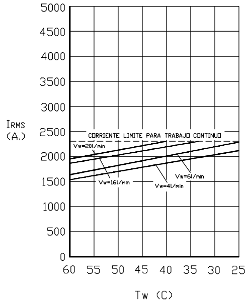
Corriente I_{RMS} máxima en trabajo continuo.
