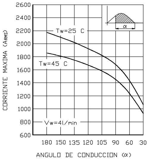
Corriente I_{RMS} máxima según el ciclo de trabajo.
