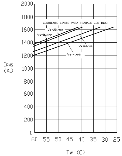
Corriente I_{RMS} máxima en trabajo continuo.
