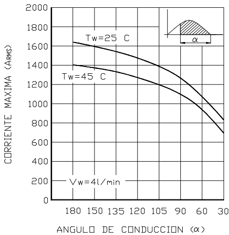
Corriente máxima / ángulo de conducción.
