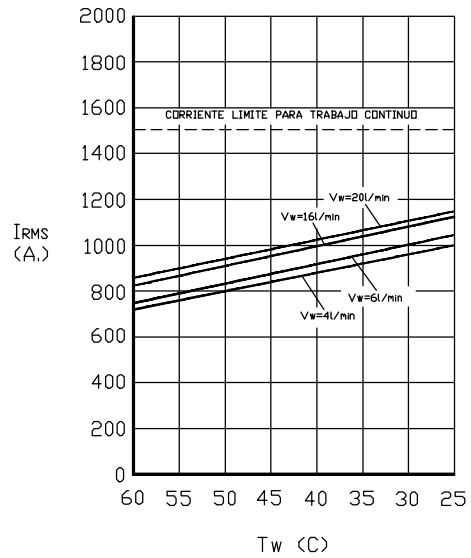
Corriente I_{RMS} máxima en trabajo continuo.
