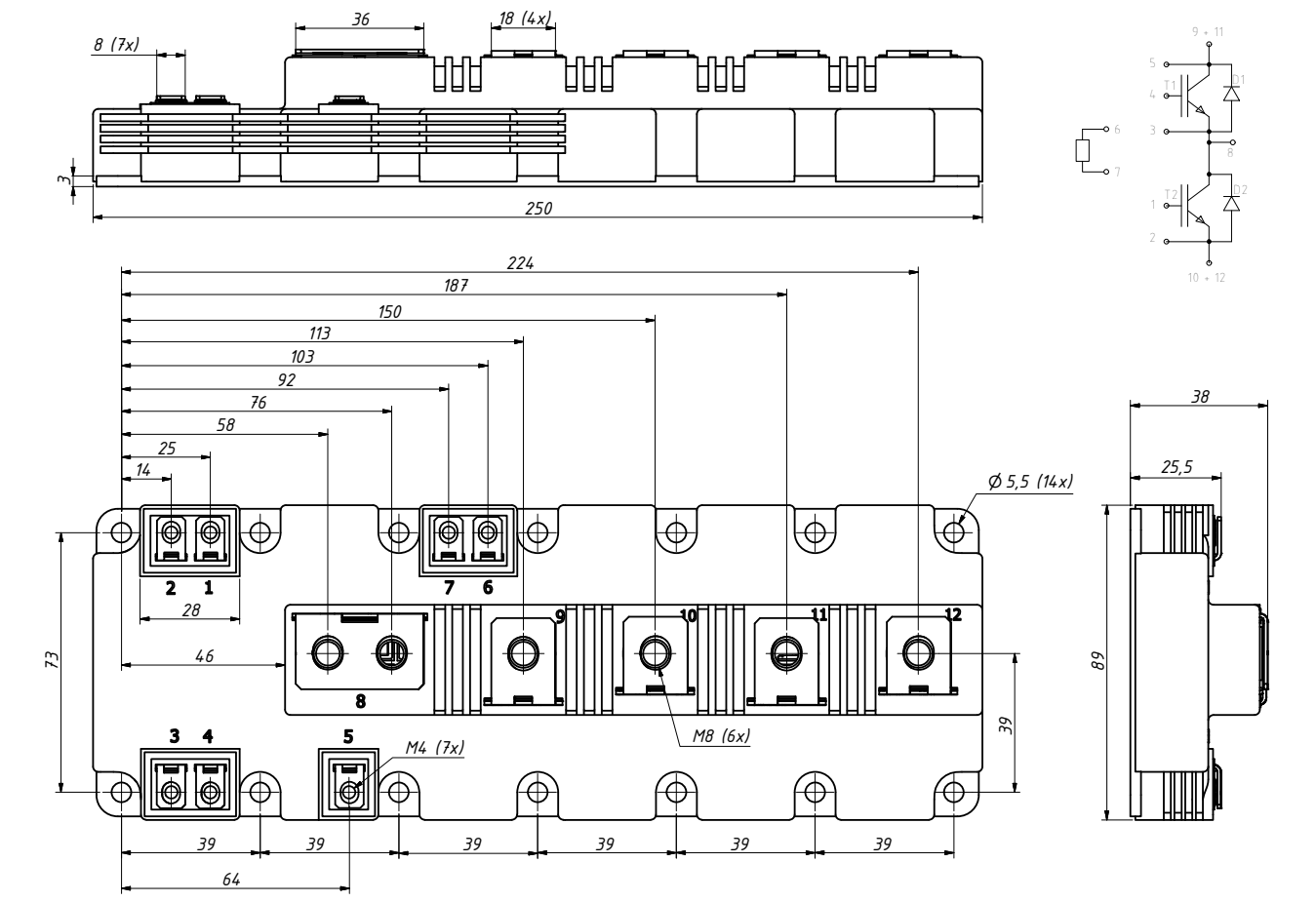
X144 SimBus P
