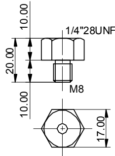
ADP1/4-M8
