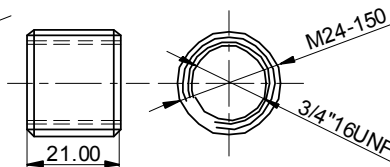
ADP3/4-M24
