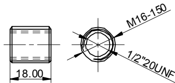
ADP1/2-M16
