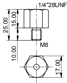
ADP1/4-M8L
